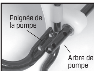
Figure 2 Alignez les trous
