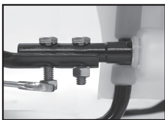
Figure 4 Apriete las tuercas a los pernos
